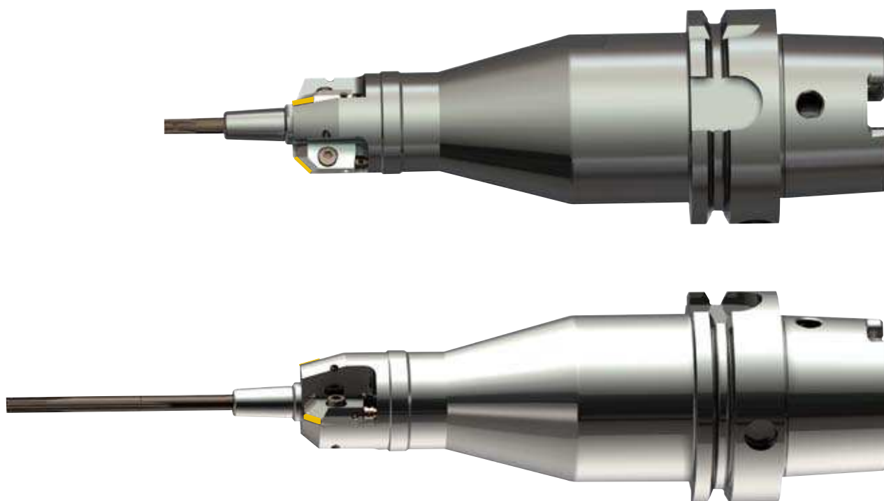
Пример: инструмент для обработки седла клапана с использованием пластин Fullface
